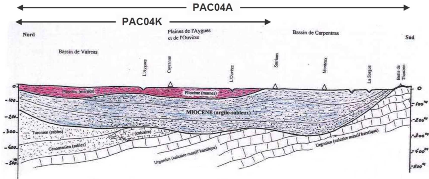
Coupe à travers le Comtat Venaissin (CPE_55), d'après Bel, 1998
