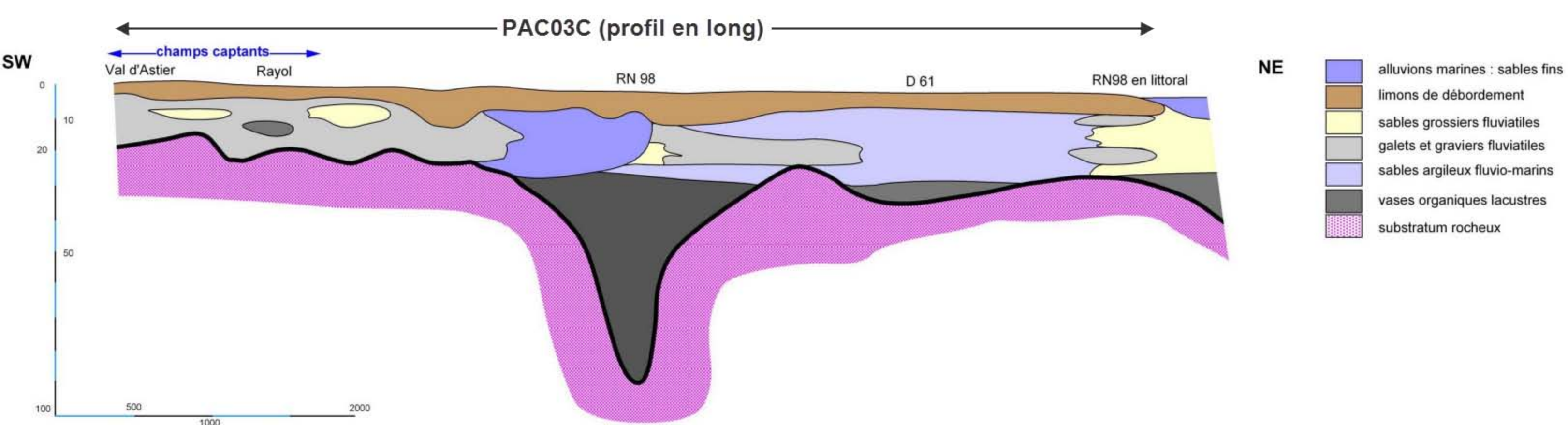
PROFIL LITHOLOGIQUE DU LITTORAL AUX CAPTAGES DE LA MOLE
