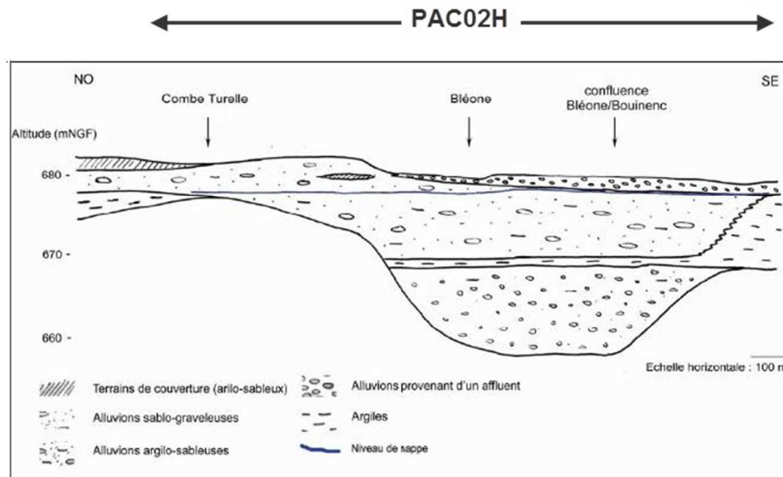
Coupe géologique interprétative entre la Combe Turrelle et la confluence Bléone/Bouinenc
