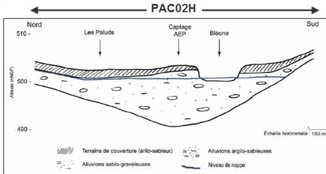
Coupe géologique interprétative du secteur de Mallemoisson
