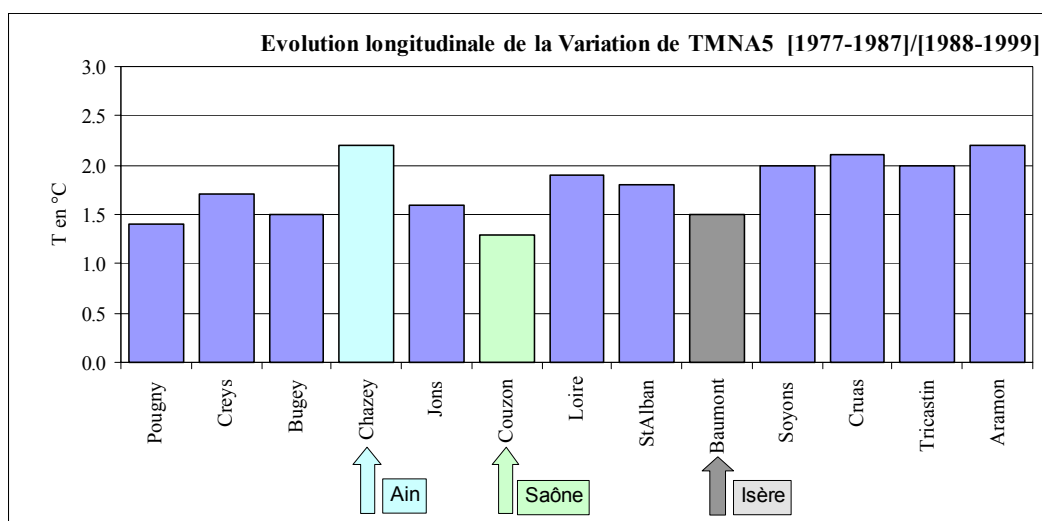
Figure 9 : évolution longitudinale de la variation de TMNA5 [1977-1987]/[1988-1999]
