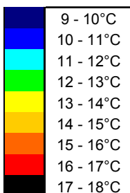
Figure 11 : représentation cartographique des températures moyennes annuelles par année et par station.
