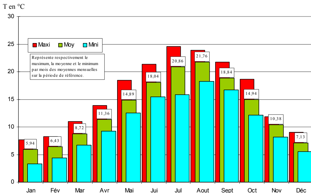
Figure 12 : régime annuel à Saint Alban (1977-1999)
