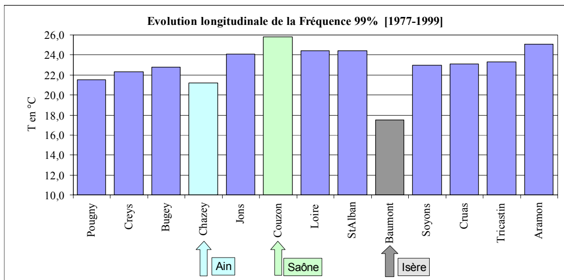
Figure 16 : évolution de la fréquence 99 % [1977 - 1999]
