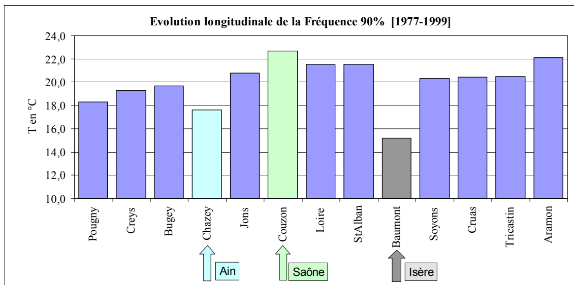
Figure 15 : évolution de la fréquence 90 % [1977 - 1999]
